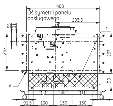
Widok z góry, wersja 4-biegunowa
