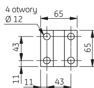
Wersja S, N & H
