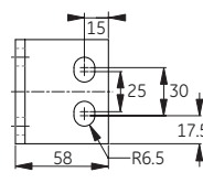
Wersja S - grubość 12 mm
