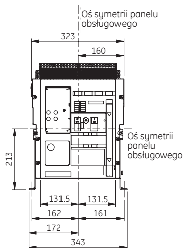
Otwór w drzwiach
