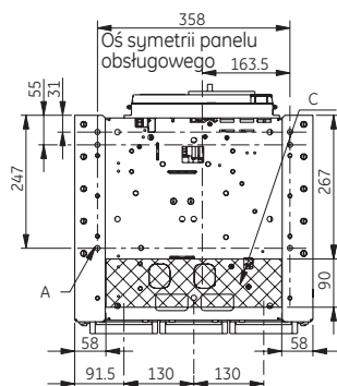
Widok z góry, wersja 3-biegunowa
