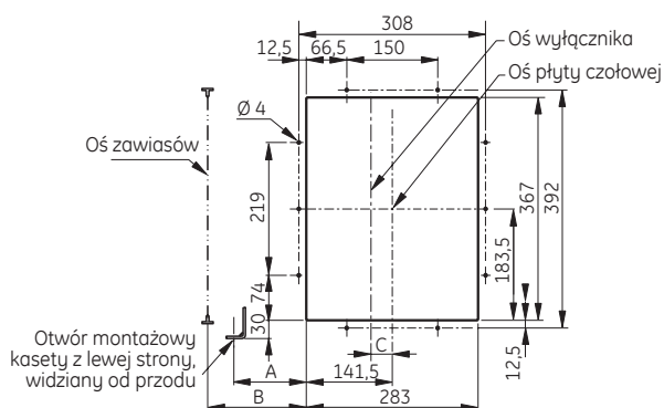
Otwór w drzwiach
