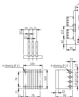
Przyłącza uniwersalne tylko pionowe maks. 4000 A
