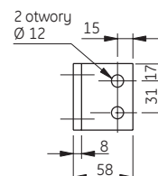
Wersja N & H - grubość 20 mm
