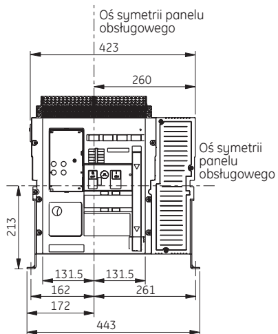
Widok z przodu, wersja 4-biegunowa
