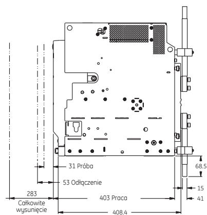
Wersja wysuwna, przyłącza z przodu Widok z boku
