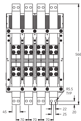
Wersja wysuwna, przyłącza z przodu wersja 4-biegunowa
