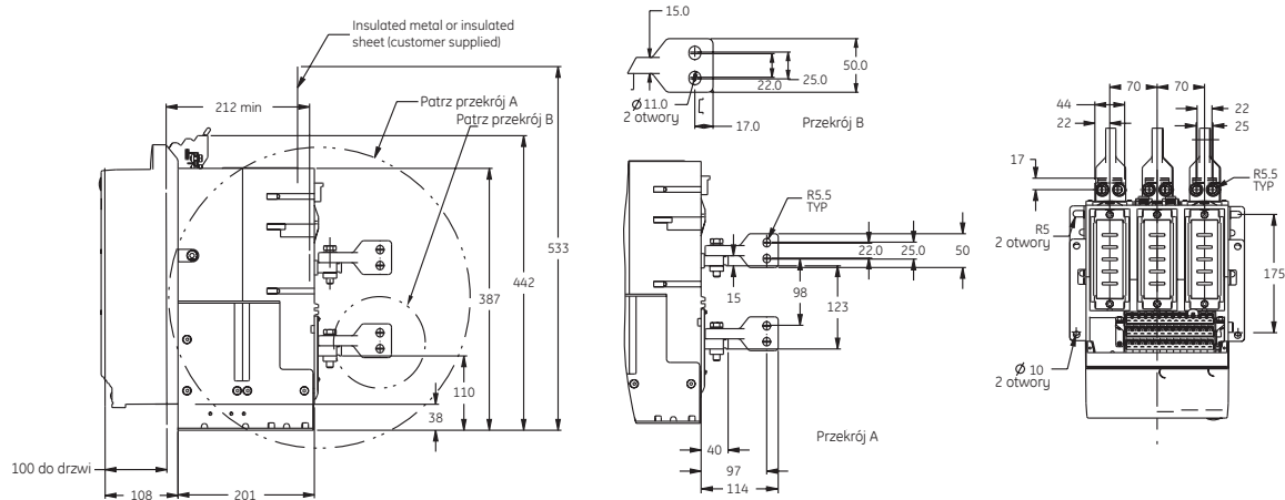
Wersja stacjonarna, przyłącza pionowe z tyłu
