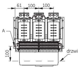
Widok z góry, wersja 3-biegunowa
