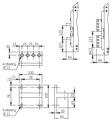
Przyłącza uniwersalne pionowe lub poziome maks. 3200 A
