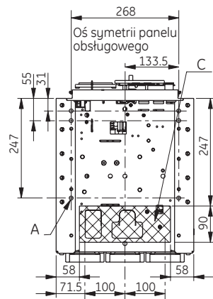
Przyłącza uniwersalne zamontowane poziomo lub pionowo
