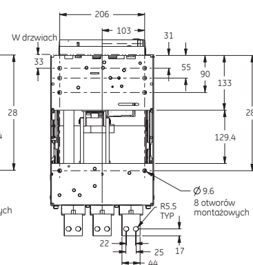
Widok z dołu, wersja 3-biegunowa
