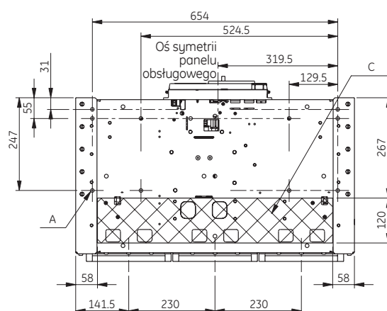
Widok z góry, wersja 3-biegunowa
