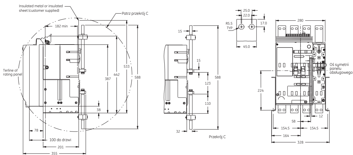
Wersja wysuwna, przyłącza z przodu wersja 4-biegunowa
