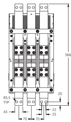
Wersja wysuwna, przyłącza z przodu wersja 3-biegunowa
