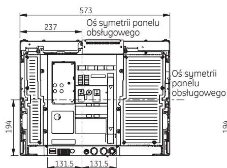
Widok z góry, wersja 4-biegunowa
