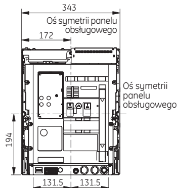
Widok z przodu, wersja 3-biegunowa
