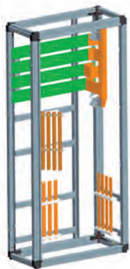
Szyny płaskie mocowane z tyłu, do 1600A
