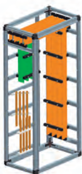
Szyny płaskie mocowane z tyłu, do 2000A
